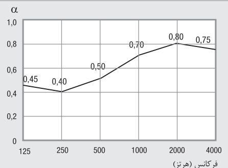
با عایق پشم سنگ
