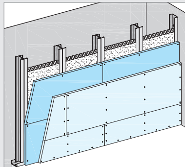
FR (25 + 18) W628 F(60)
